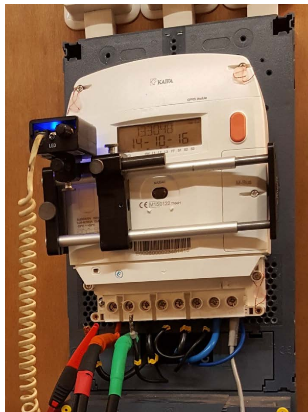
Testopstelling onderzoek elektriciteitsmeter
